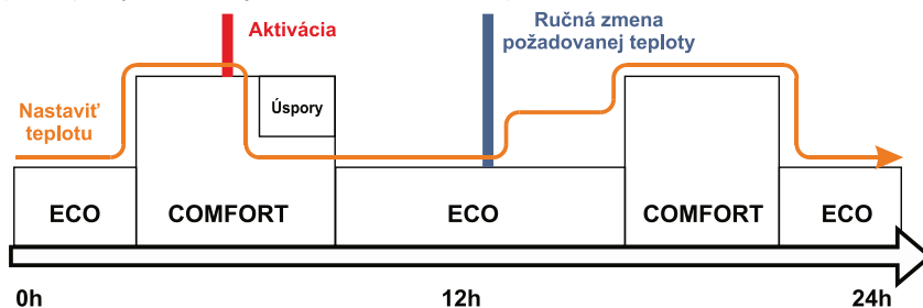
Obr. 6: Vývoj teploty pre jednotlivé činnosti systému
