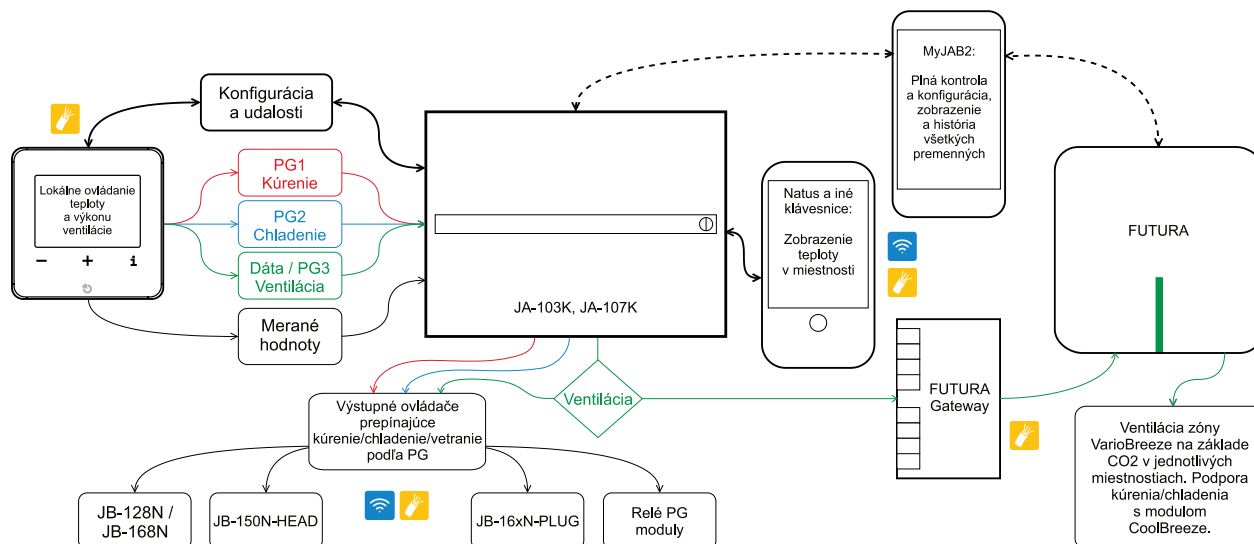
Obr. 4: Všeobecná konfigurácia riadenia HVAC.
