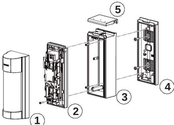
Obr. 1.: 1 - horný kryt, 2 - základná doska detektora, 3 - zadný kryt, 4 - montážna podložka, 5 - strieška zadného krytu
