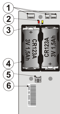
Obr. 3 - Rádiový vysielač JA-150TX-VXi: 1 – konektor pre prepájanie s detektorom, 2 – červená kontrolka aktivácie PIR, 3 – žltá kontrolka aktivácie Antimaskingu a vybitých batérií, 4 – držiak batérií, 5 – konektor pre pripojenie externej antény AN-868, 6 – sériové číslo
