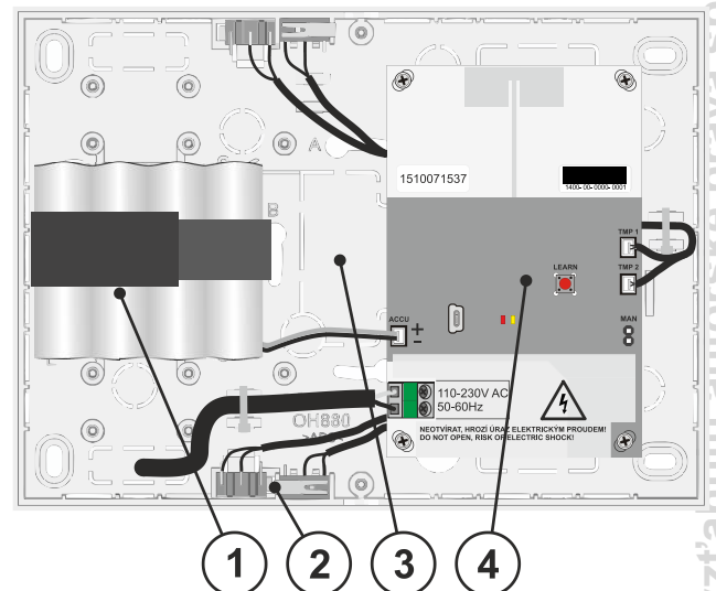
Obr. 2: 1 – zálohovací akumulátor; 2 – sabotážne kontakty; 3 – zadná časť plastu; 4 – elektronika (modul)
